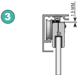
SE HA DE RESPETAR LA COTA DE 1,5 MM. PARA EVITAR QUE EL TOPE INTERCEDA CON LA MORDAZA.
