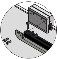
DETALLE FIJACIÓN A SOPORTE.
