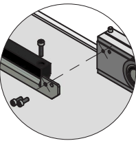
DETALLE FIJACIÓN A MORDAZA.
