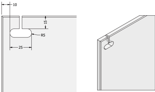
MECANIZADO PARA VIDRIO FIJO LATERAL PARA USAR LA PIEZA CORNER LATERAL
