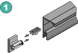
COLOCACIÓN DE TOPE FRENO Y TOPE SOFTCLOSE DENTRO DEL PERFIL GUÍA ANTES DE LA INSTALACIÓN EN OBRA.
